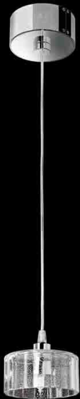
170/1S Diamond Chrome Ø 12 cm - h. 50-150 cm - Kg. 1,5 1 x G9 halopin max 40Watt
